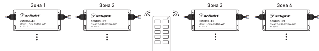
Рисунок 3. Вариант построения системы с 4-зонным пультом дистанционного управления
