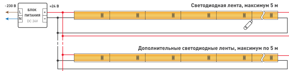
Схема 1. Подключение нескольких светодиодных лент с двух сторон Рекомендуется использовать для обеспечения равномерного свечения ленты по всей длине.
