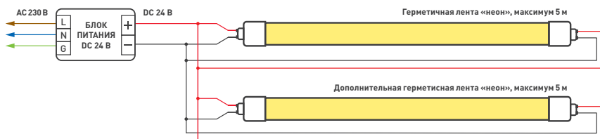
Схема 1. Подключение нескольких герметичных лент «неон»
