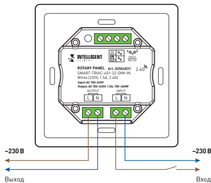
Рис. 1. Типовая схема подключения панели
